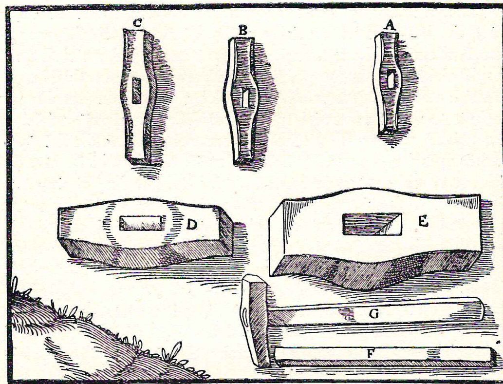
Zásekový mlátek A. Mlátek B. Pucka C. Dvouruční pucka D. Perlík E. Dřevěné topůrko F. Topůrko v zásekovém mlátku G.
