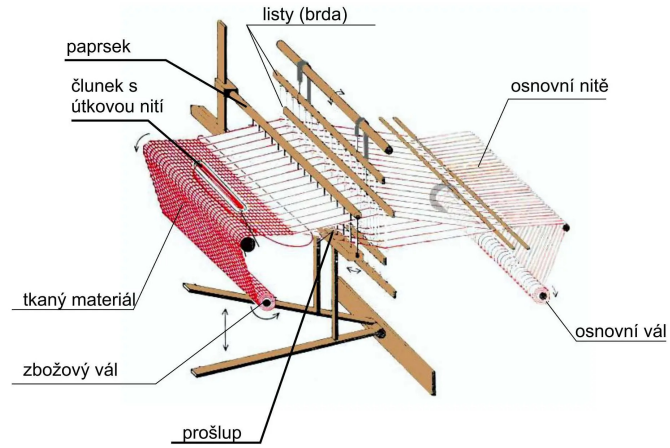
TKACÍ STAV
