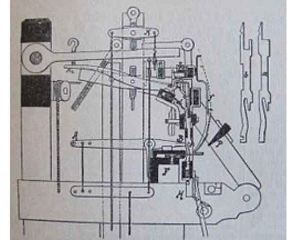
PLETACÍ STÁVEK
